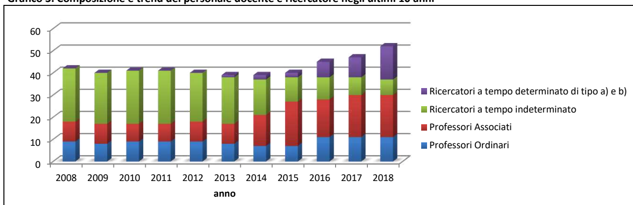
Grafico 3. Composizione e trend del personale docente e ricercatore negli ultimi 10 anni
