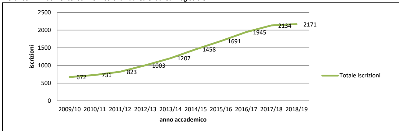
Grafico 2. Andamento iscrizioni corsi di laurea e laurea magistrale
